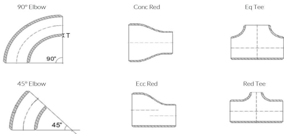
ASME B36.19/ASME B36.10 Unit : mm
