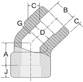
45° Elbow
